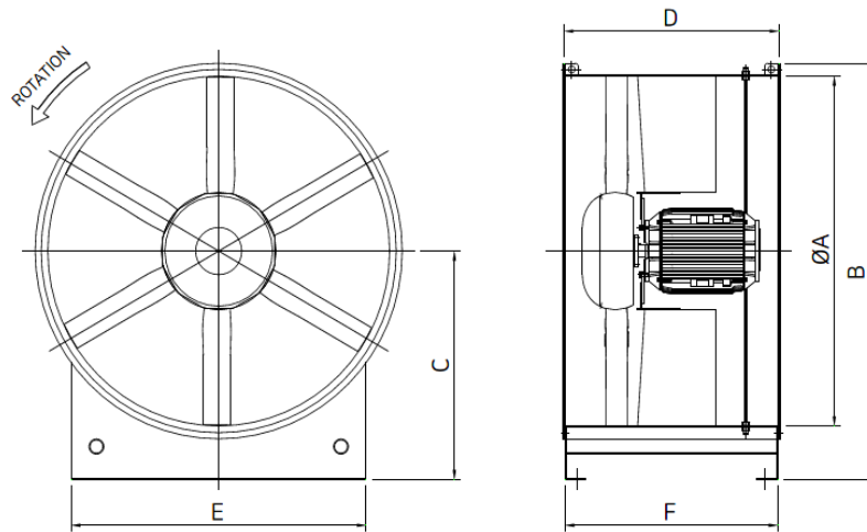
DIMENSION(mm)
