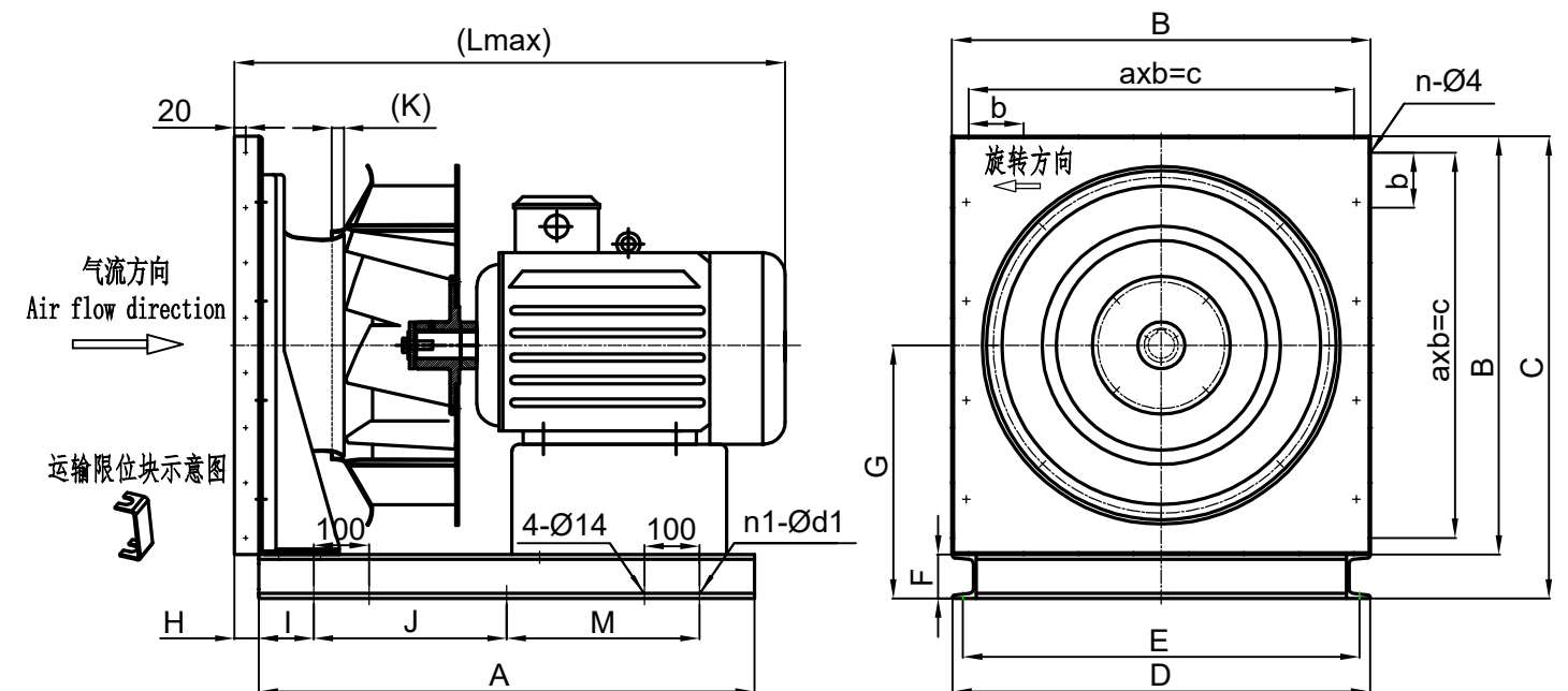
YPFA 系列风机外形尺寸
