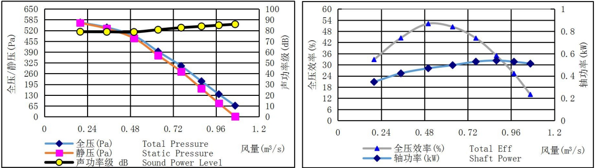
HTFC-255-10 转速(Speed): 2600r/min
