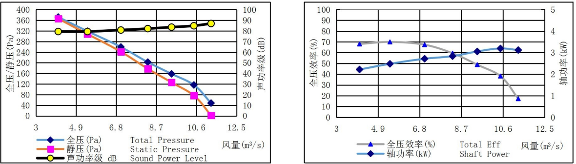
HTFC-900-12 转速(Speed): 700r/min FEG71
