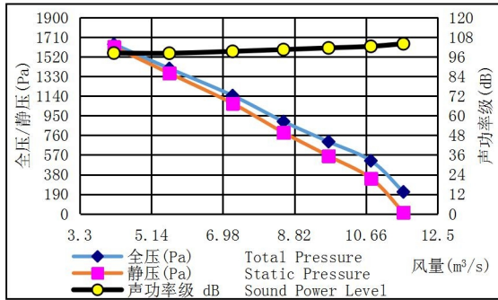
HTFC-710-12 转速(Speed): 600r/min
