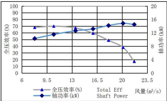
HTFC-1000-12 转速(Speed): 900r/min FEG71
