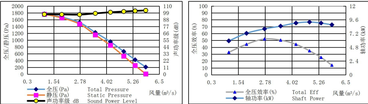
HTFC-450-10 转速(Speed): 2400r/min
