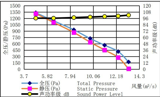
HTFC-710-12 转速(Speed): 1400r/min
