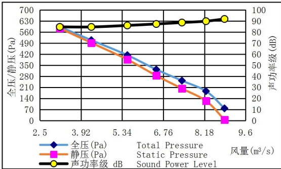
HTFC-710-12 转速(Speed): 1000r/min
