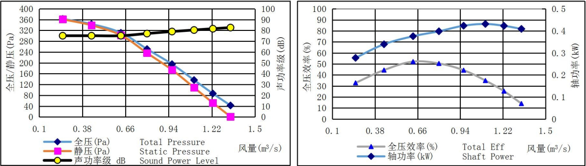
HTFC-320-10 转速(Speed): 1600r/min
