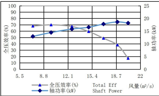
HTFC-900-12 转速(Speed): 1100r/min FEG71
