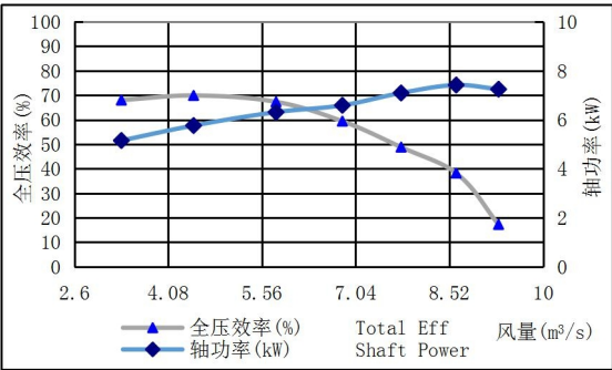
HTFC-630-12 转速(Speed): 1300r/min
