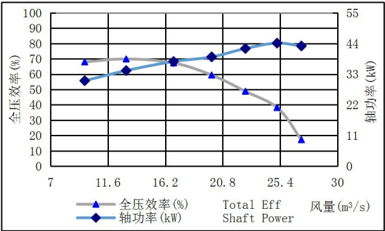
HTFC-1000-12 转速(Speed): 500r/min FEG71
