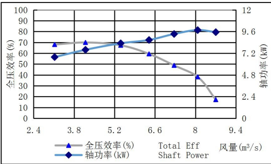
HTFC-560-12 转速(Speed): 1800r/min
