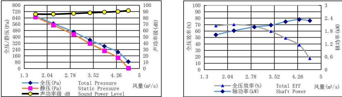
HTFC-500-12 转速(Speed): 1400r/min
