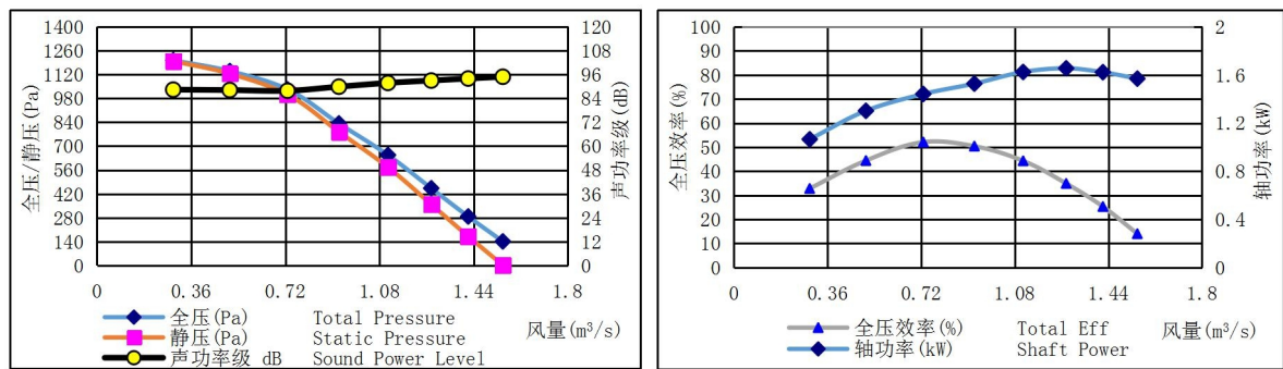
HTFC-255-10 转速(Speed): 3500r/min
