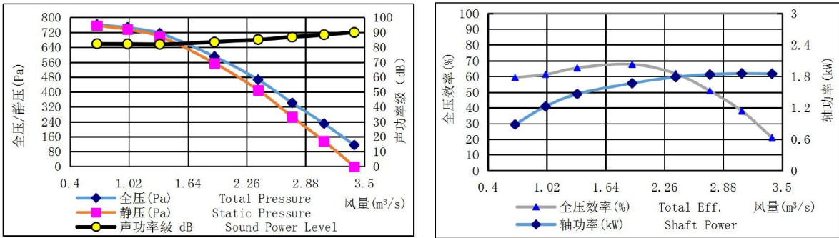
HTFC-400-10 转速(Speed): 2000r/min
