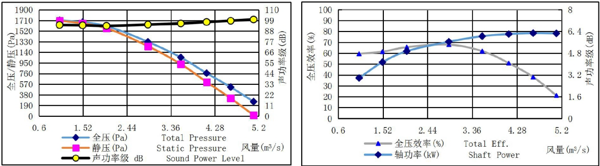
HTFC-400-10 转速(Speed): 2800r/min
