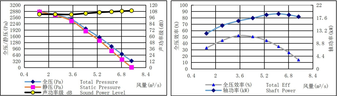
HTFC-500-12 转速(Speed): 900r/min
