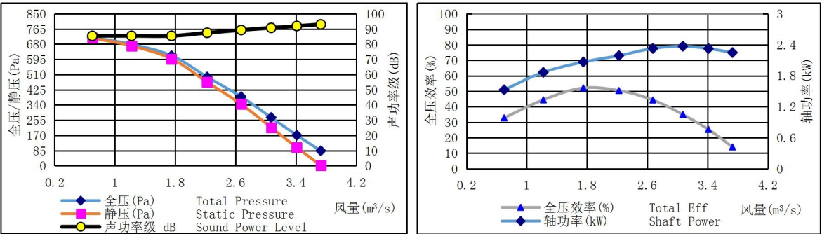
HTFC-450-10 转速(Speed): 1800r/min
