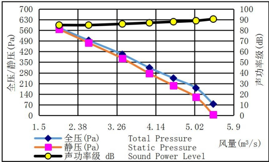
HTFC-560-12 转速(Speed): 1200r/min
