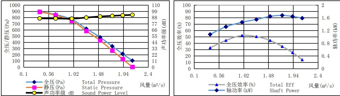
HTFC-320-10 转速(Speed): 2600r/min
