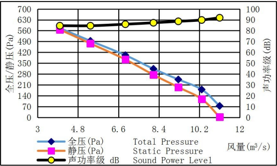
HTFC-800-12 转速(Speed): 900r/min
