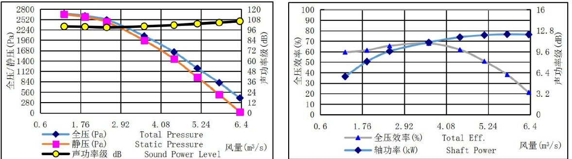
HTFC-450-10 转速(Speed): 1000r/min
