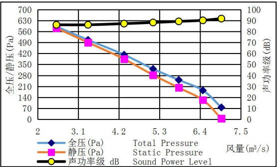
HTFC-630-12 转速(Speed): 1100r/min
