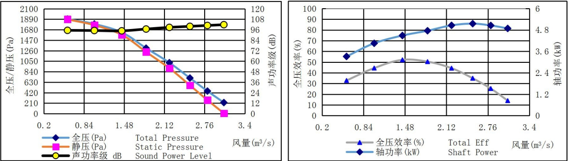
HTFC-320-10 转速(Speed): 3500r/min
