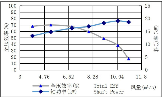
HTFC-630-12 转速(Speed): 700r/min
