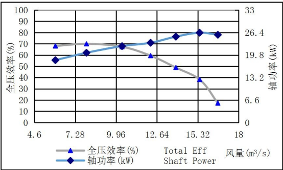
HTFC-800-12 转速(Speed): 500r/min
