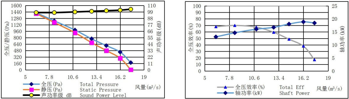
HTFC-800-12 转速(Speed): 1300r/min FEG71
