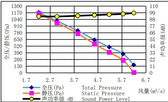
HTFC-500-12 转速(Speed): 2000r/min
