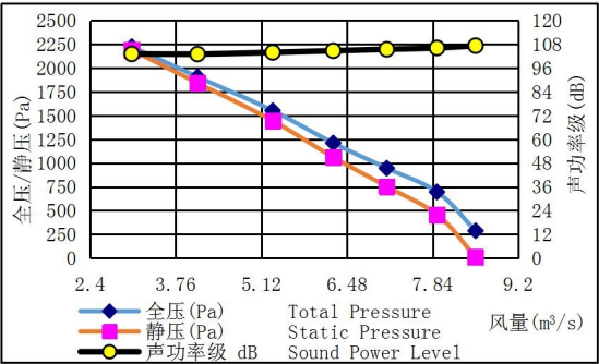
HTFC-560-12 转速(Speed): 800r/min
