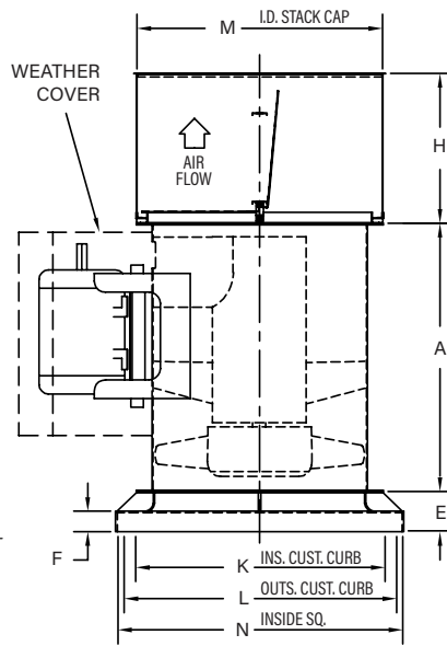
ARR. 9 - ROOF VENTILATOR
