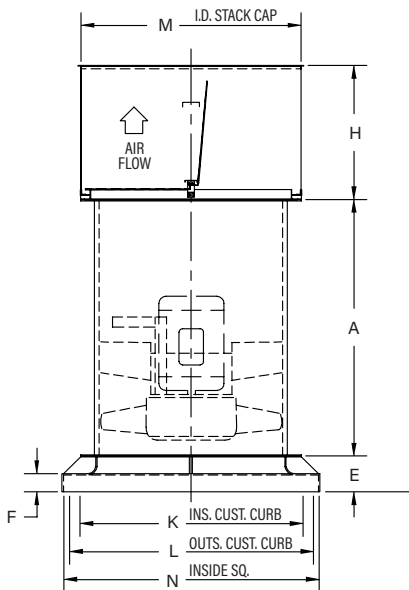
ARR. 4 - ROOF VENTILATOR
