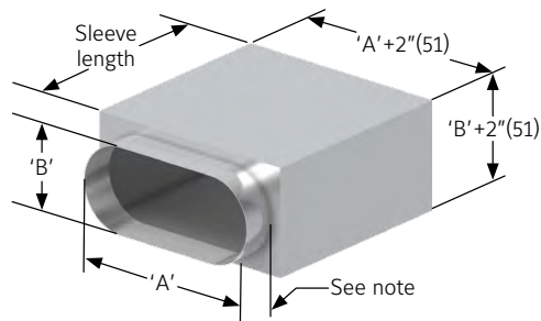
FSD37 STYLE LO, CO & WO FSD37LP STYLE LO & CO
