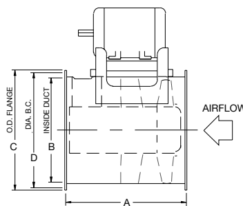
ARR. 9 - HORIZONTAL
