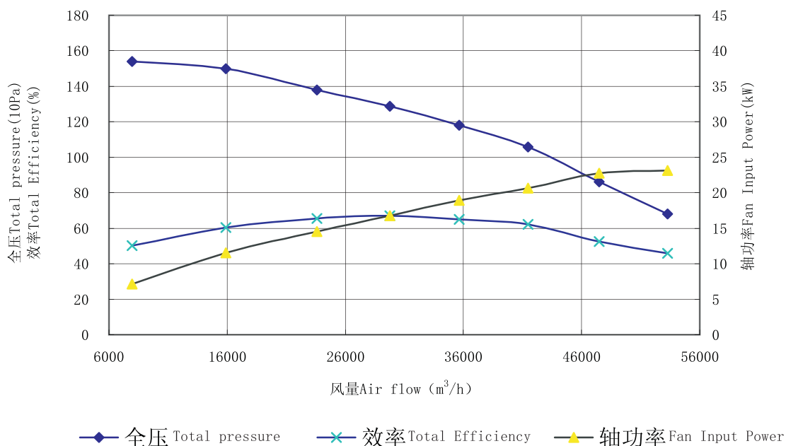
4-79-10E性能曲线图 (Performance curve) n=1000\text{r/min}
