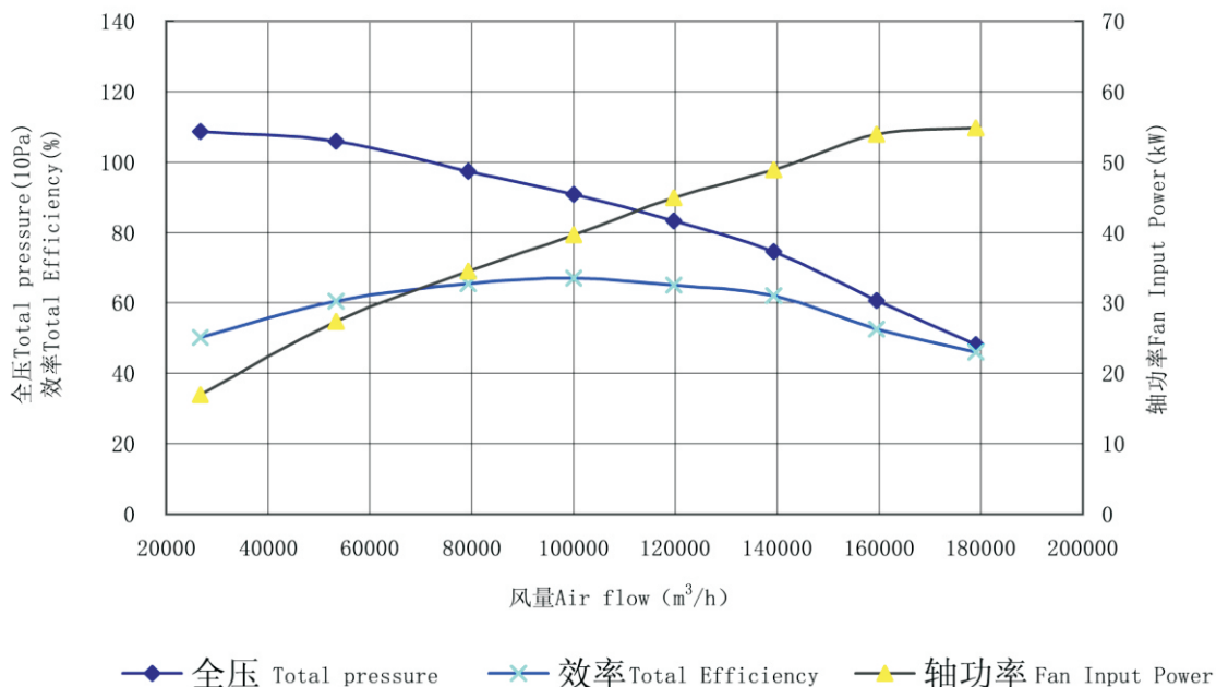
4-79-20E性能曲线图 (Performance curve) n=420\text{r/min}
